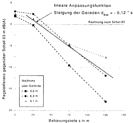
Bild 3: Meßquerschnitt 2, B = 0,12 , h_B = 10 m, ohne Schallschutz
