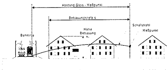
Bild 2: Prinzipdarstellung der mittleren Bebauungshöhe h_B , der Bebauungstiefe s sowie des Schallweges durch die Bebauung
