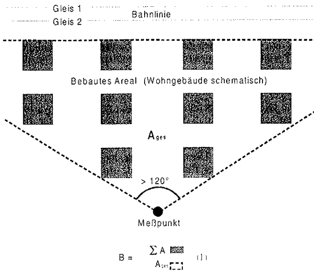
Bild 1: schematische Darstellung der Bebauungsdichte B
